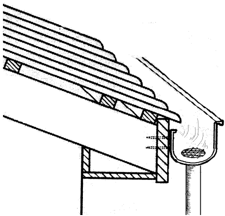
Figure 24 : Filtre grossier
